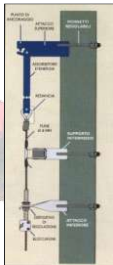
Sistema anticaduta per tralicci
